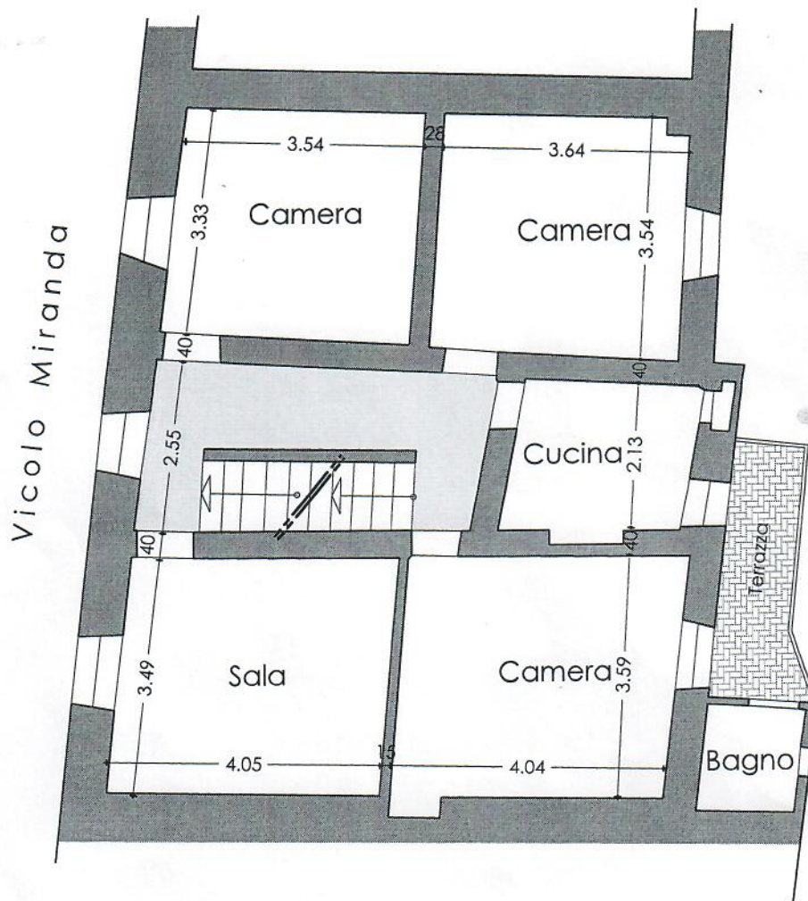
PIANO PRIMO
